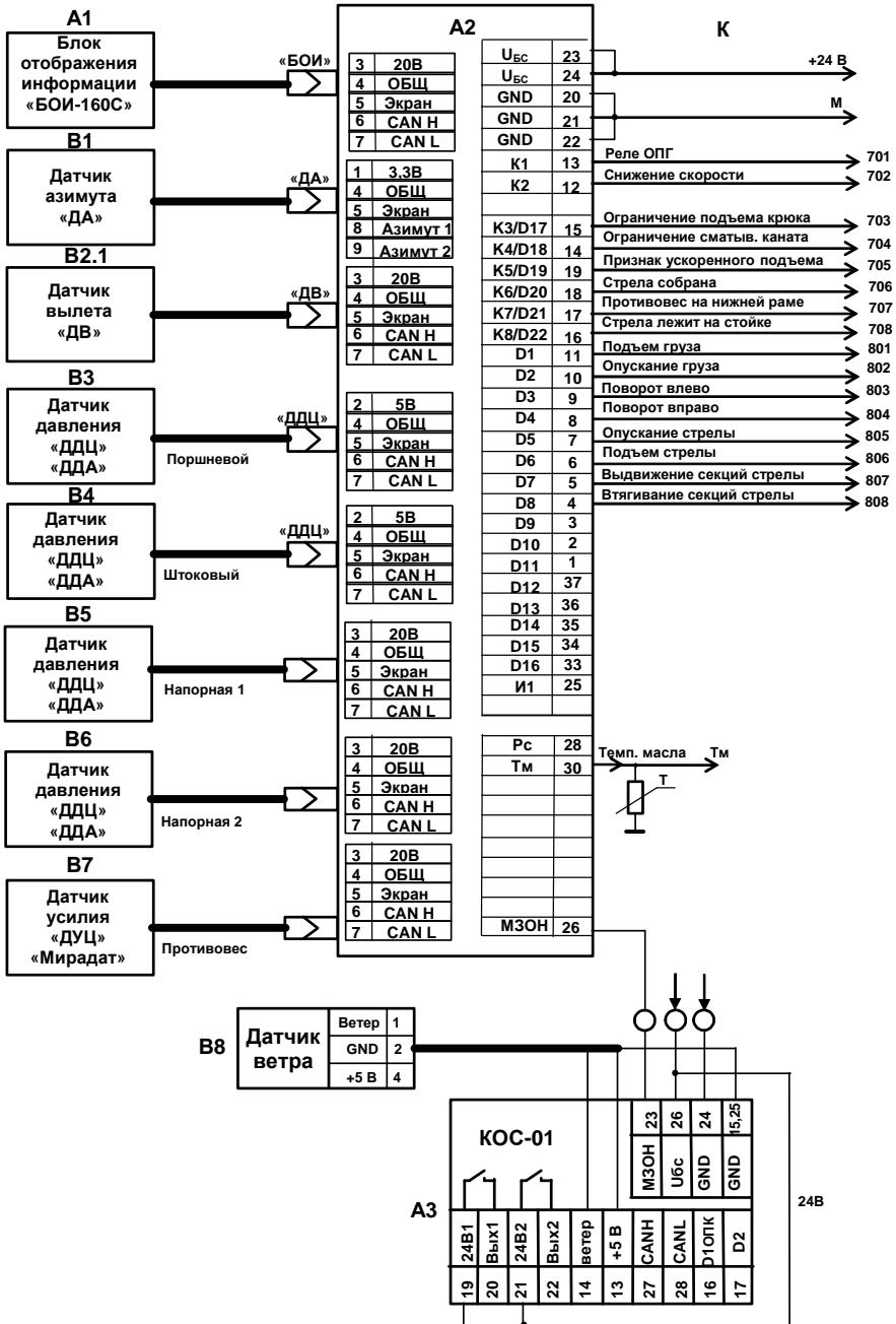
Рисунок Б.10 – Схема подключения ОНК-160С-24, - 144 на кране
