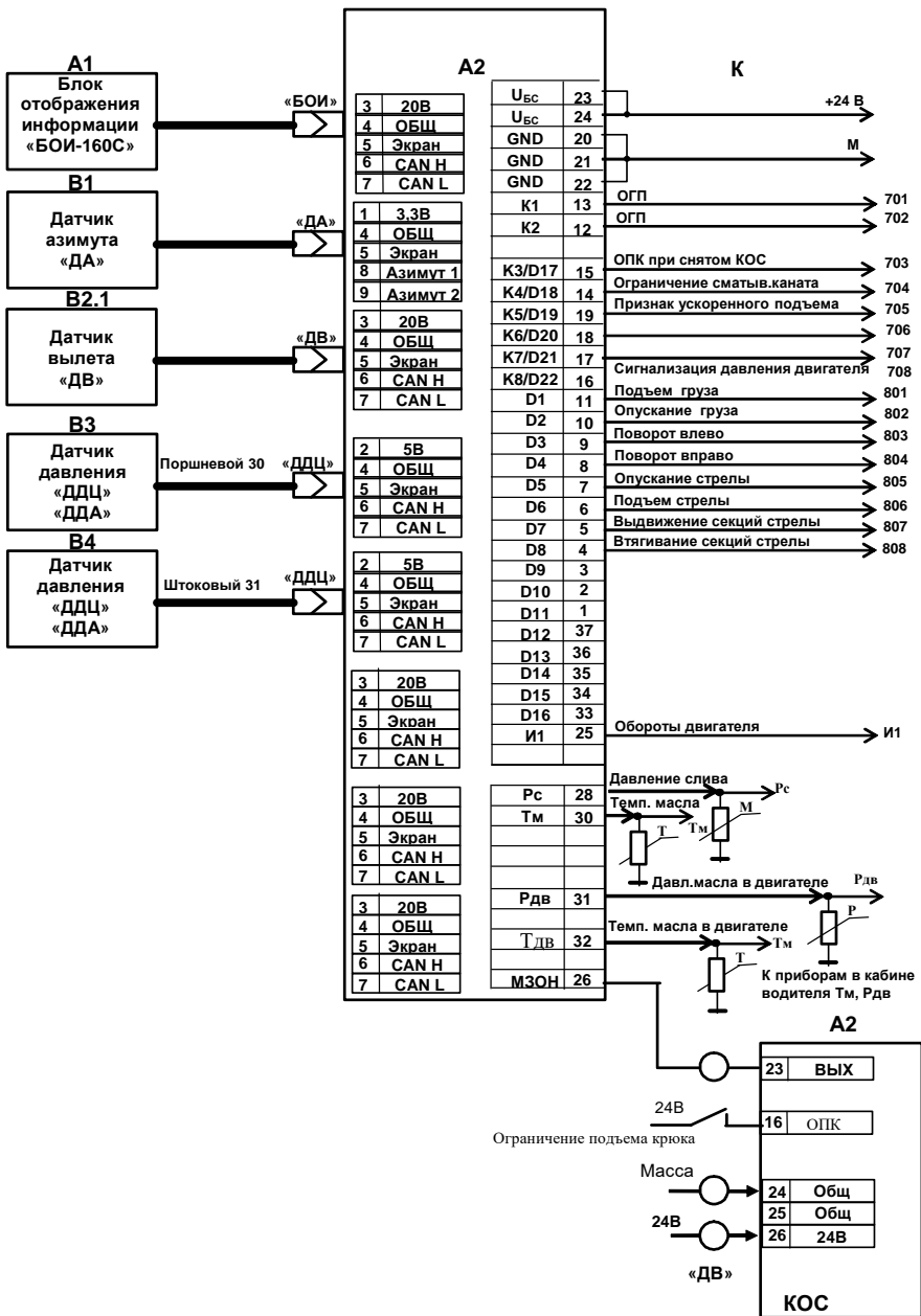
Рисунок Б.10.1 – Схема включения ОНК-160С-53, -79, -108 на кране
