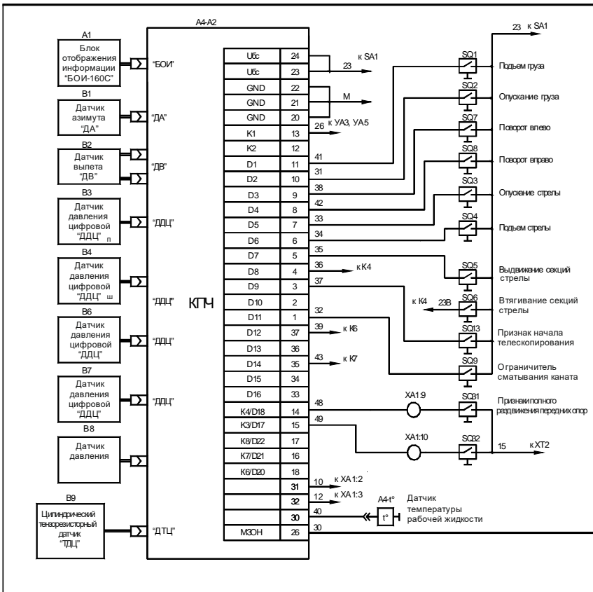
Рисунок Б.12 – Схема подключения ОНК-160С-55.01 на кране КС-65713-5
