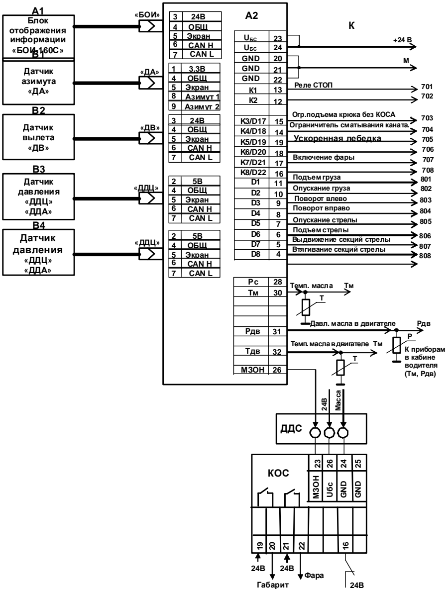
Рисунок Б.11 – Схема подключения ОНК-160С-54 на кране КС-55726; ОНК-160С-109 на кране
